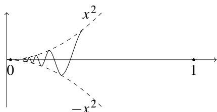
Funkce F .
