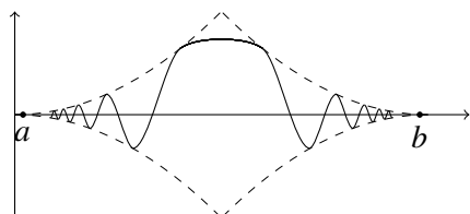
Funkce F_{a,b}
